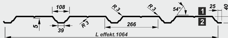
WAND -/ KONSTRUKTIONSPROFIL
