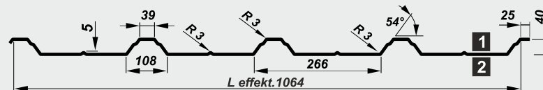
DACHPROFIL
